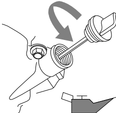
Figure 4-10. Remplissage d'huile moteur
