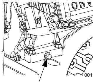
Figure 4-12. Bouchon de vidange d'huile
