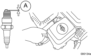
000134a Figure 4-13. Bougie d'allumage
