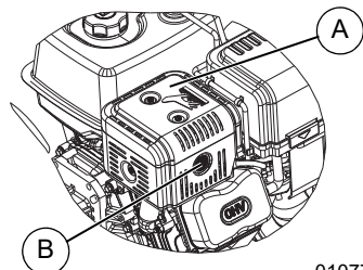
Figura 4-14. Extraer el dispositivo antichispas
