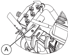
Figure 2-3. Graissage de la roue pivotante
