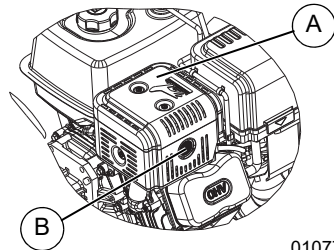
Figure 4-14. Retrait du pare-étincelles
