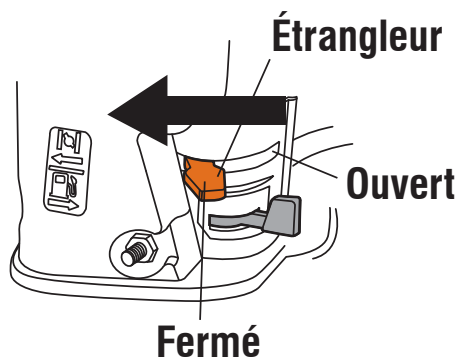
Figure 25 - Levier d'étrangleur
