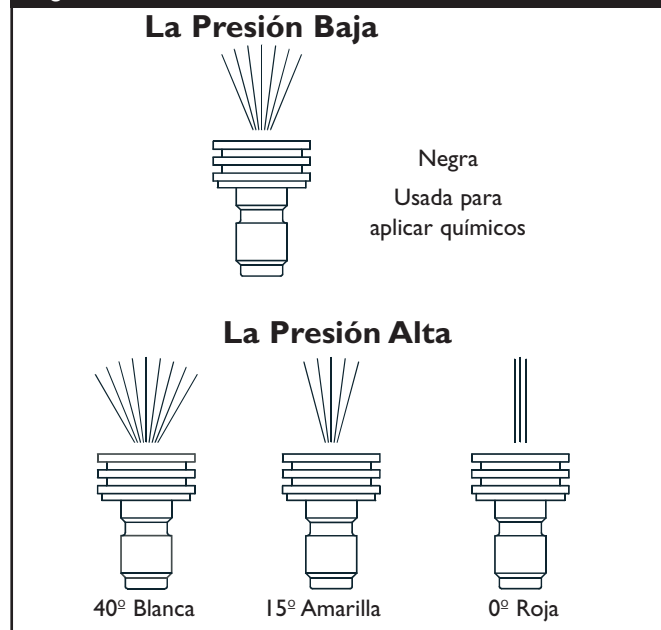
Figura 29 — Rocíe los Modelos del Rocío de Punta
